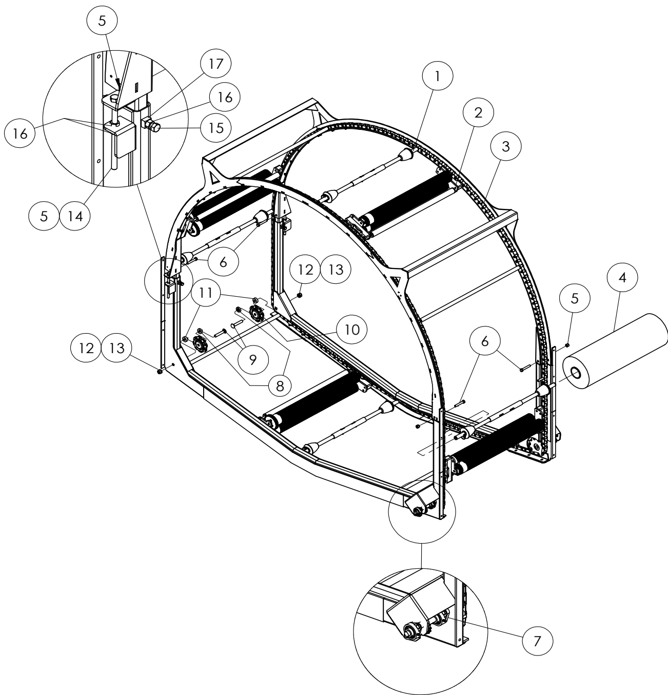
KBWA27 WRAP FRAME
